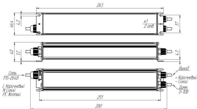
Рис. 2. Габаритный чертеж.
