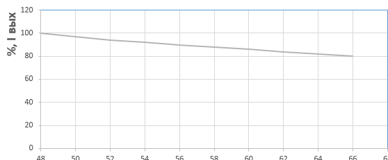
Рис.1 – График зависимости выходного тока от внешней температуры**. (При установке источника питания в горизонтальном положении на основание.)
