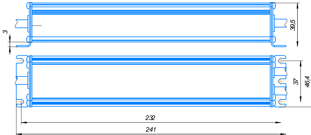
Рис. 1. Габаритный чертёж
