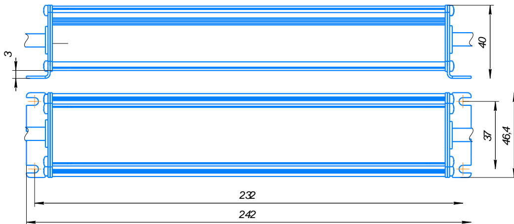
Рис. 1. Габаритный чертеж.
