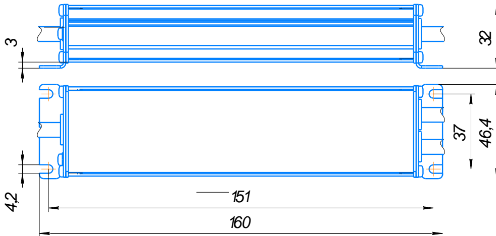
Рис. 1. Габаритный чертеж
