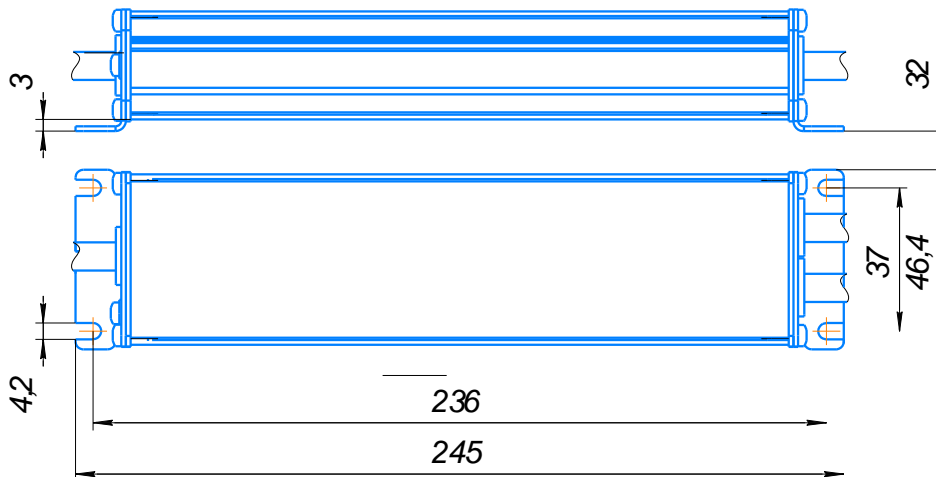
Рис. 1. Габаритный чертеж
